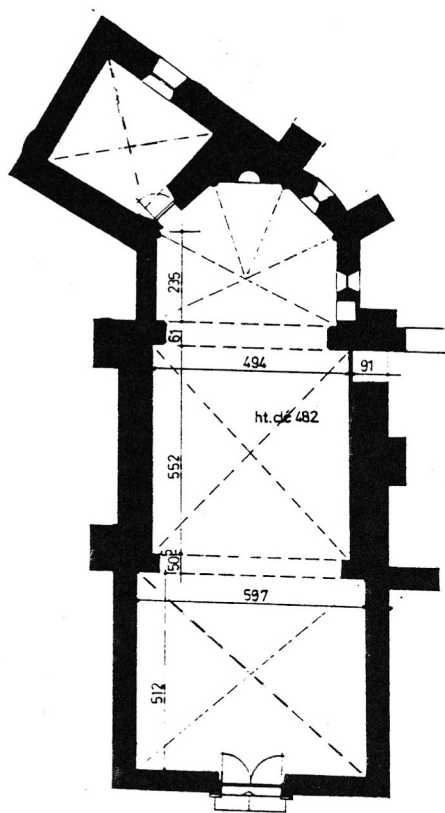
Plans de la chapelle Notre-Dame de Fougères établis par M. Marc Jean.
